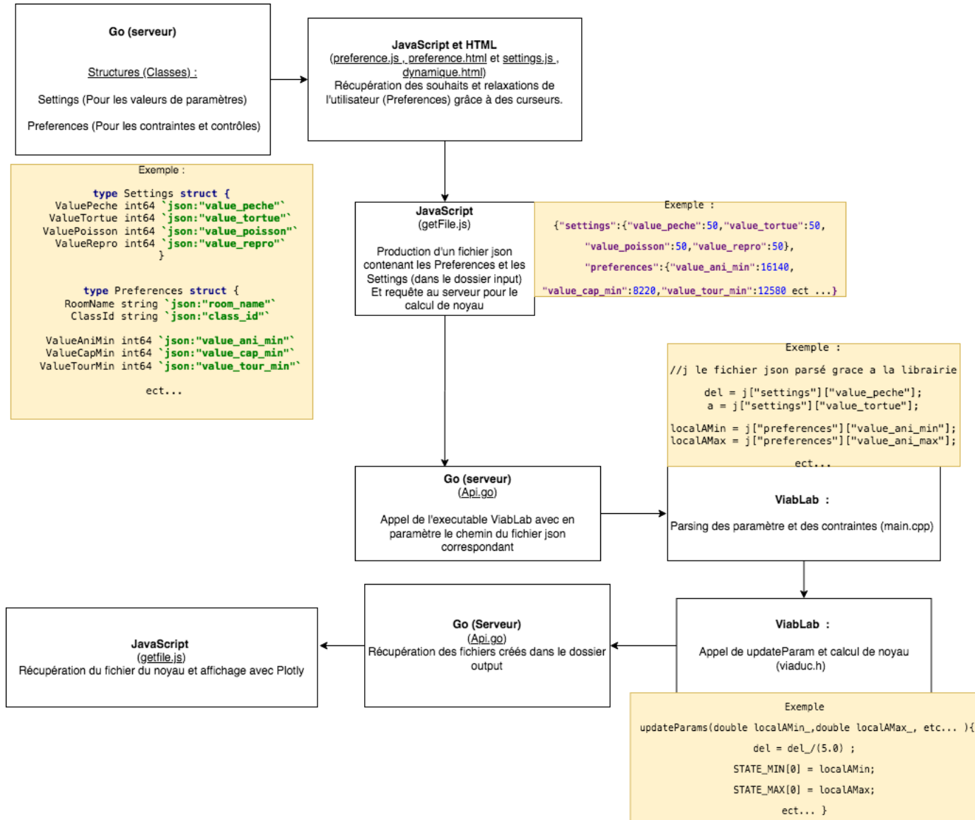
FIGURE C.1 – Fonctionnement de l'appel de ViabLab pour le calcul de noyaux dans Viaduc.
