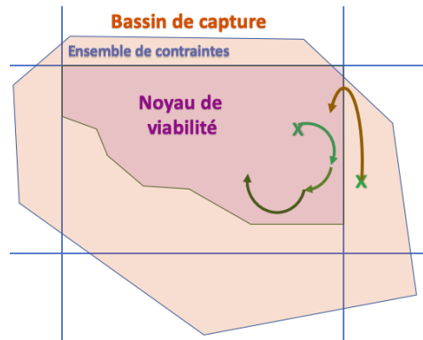
FIGURE 8.1 – Schéma du bassin de capture : les points vert appartiennent au bassin de capture et les flèches représentent les trajectoires associées à la dynamique.
