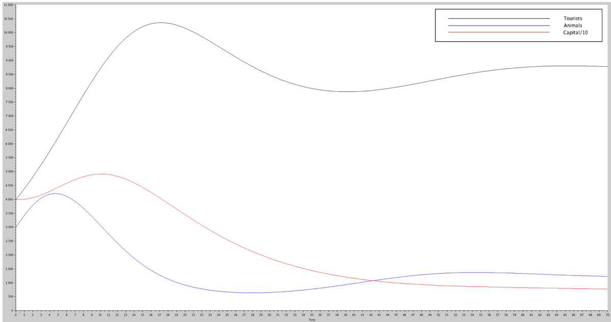
FIGURE 5.10 – A, C/10 et T en fonction du temps pour i_p = 10^{-6} et \zeta = 0.1 de t = 0 à t = 50 .
