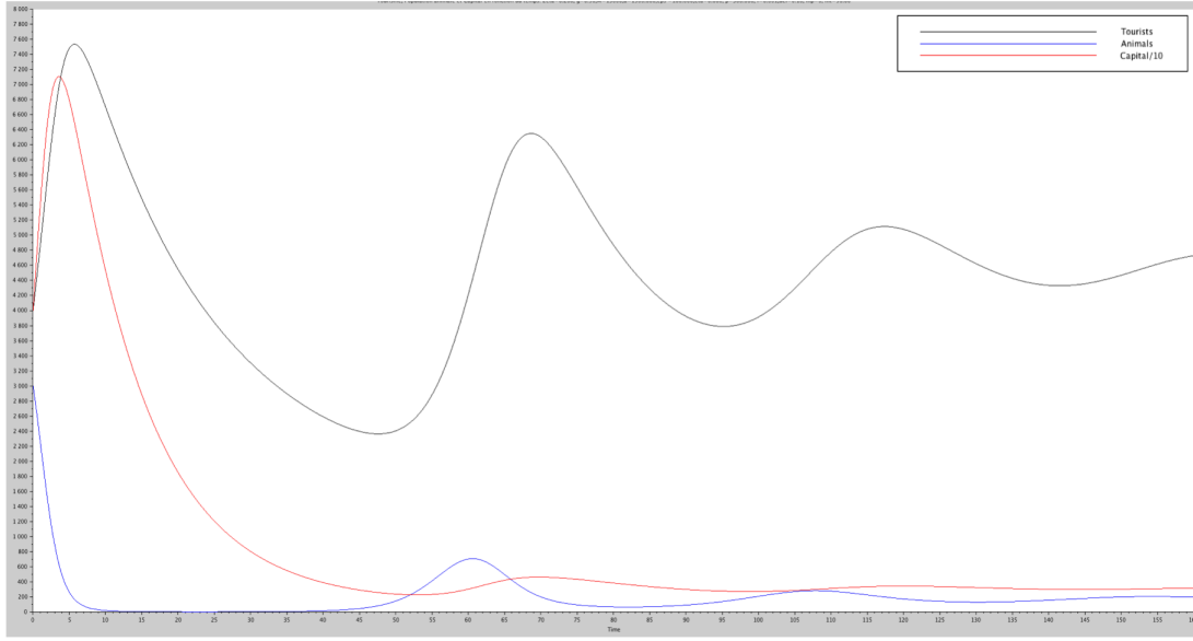
FIGURE 5.11 – A, C/10 et T en fonction du temps pour i_p = 5 \times 10^{-6} et \zeta = 0.2 de t = 0 à t = 160 .
