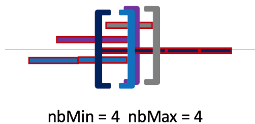
FIGURE 6.21 – L'algorithme augmente les Maxs[k] du groupe des maxima de leur valeur pasMax[k] et on diminue les Mins[k] du groupe des minima de leur valeur pasMin[k] .
