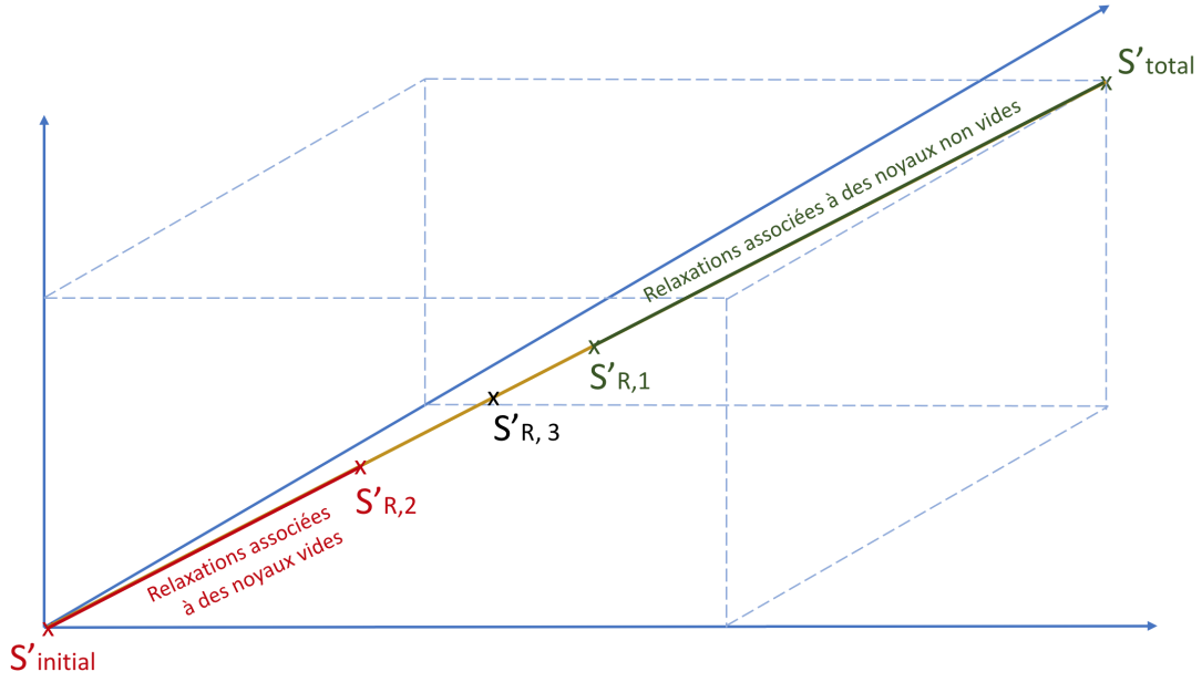
FIGURE 6.28 – Exemple de recherche dichotomique dans le cas où n = 3 et où le noyau associé à S'_{R,1} est non vide et le noyau associé à S'_{R,2} est vide.
