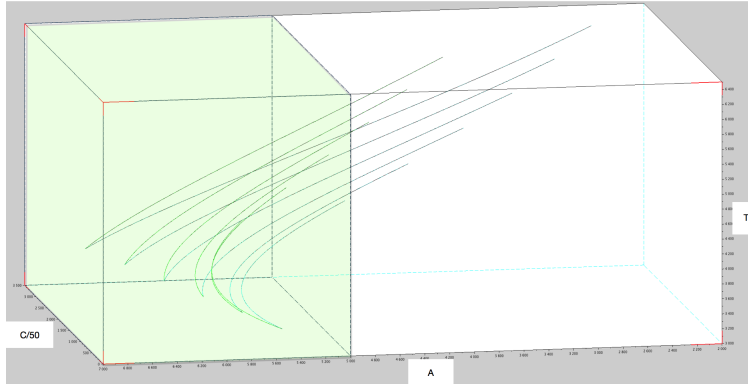
FIGURE 6.5 – Exemple de trajectoires partant de l'ensemble de contraintes du joueur (la zone verte) et utilisant les contrôles du joueur. Toutes les trajectoires calculées sortent de l'ensemble de contraintes du joueur.
