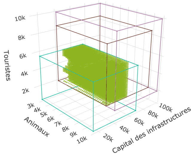
FIGURE 6.11 – Les intersections des contraintes et des contrôles des joueurs ne sont pas vides, un noyau de viabilité (en vert) a été calculé dans cette intersection. Les hyperrectangles représentent les contraintes des joueurs. Ici nous sommes dans le cas particulier où les joueurs ont la même dynamique.
