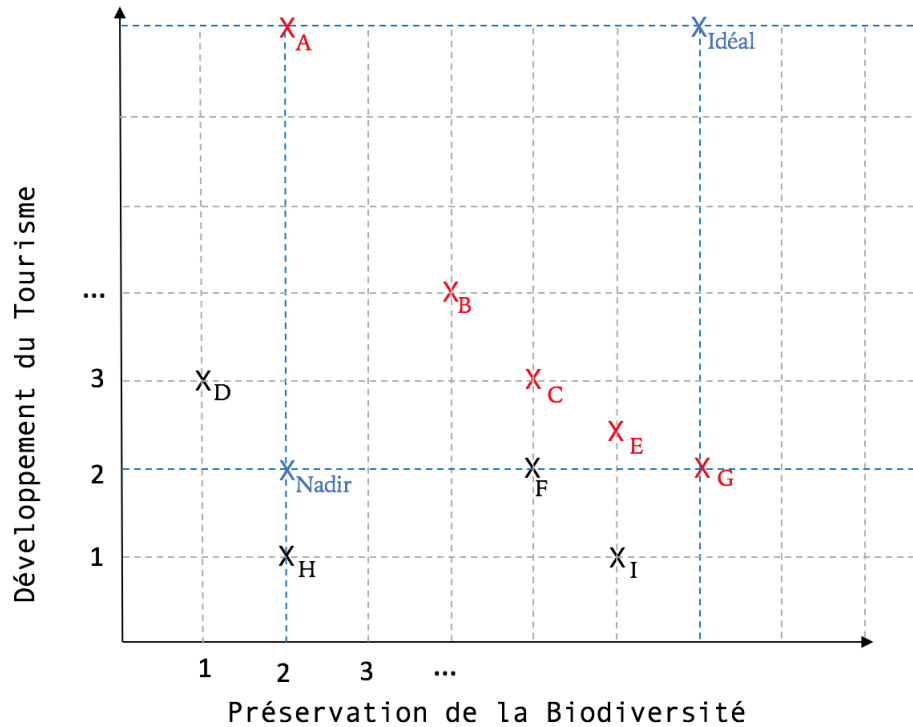
FIGURE 4.3 – Représentations des points Idéal et Nadir pour l'exemple précédent.
