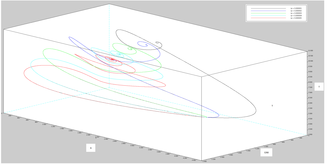
FIGURE 5.13 – Diagramme de phase de A , C/50 et T pour \zeta = 0.1 et i_p variant de 10^{-6} à 5 \times 10^{-6} .
